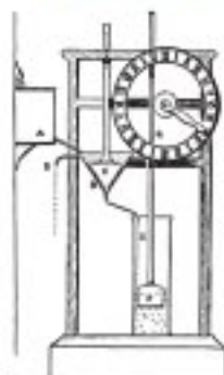
Воден часовник
